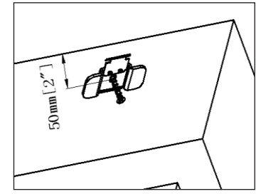
AutoWand Motorized
